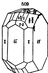
Mt. Doré.
